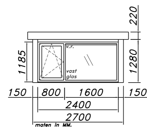
aanzicht dakkapel voorgevel
